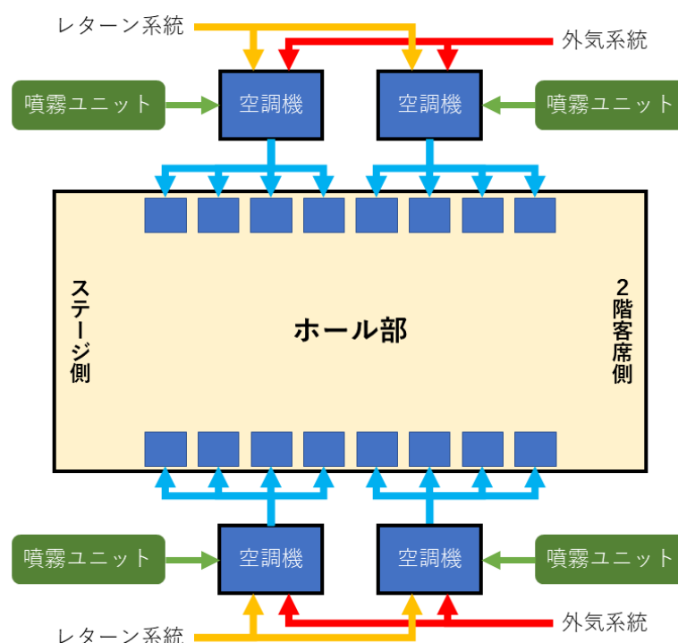
本実証実験システム概要図
