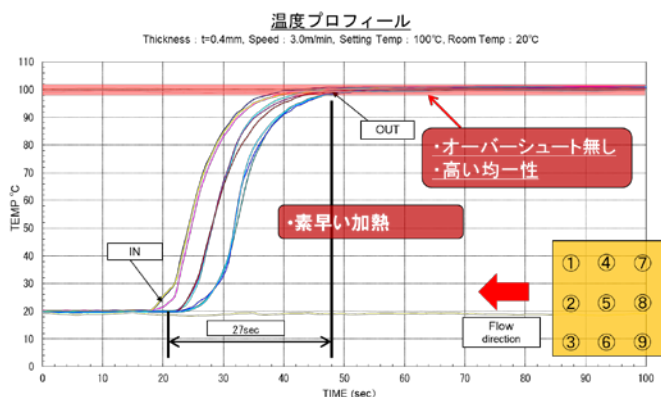
加熱時の温度プロフィール
