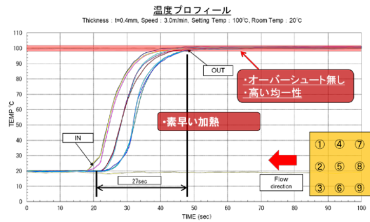
加熱時の温度プロフィール
